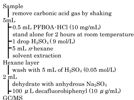
図 1 ビール中のホルムアルデヒド分析手順
